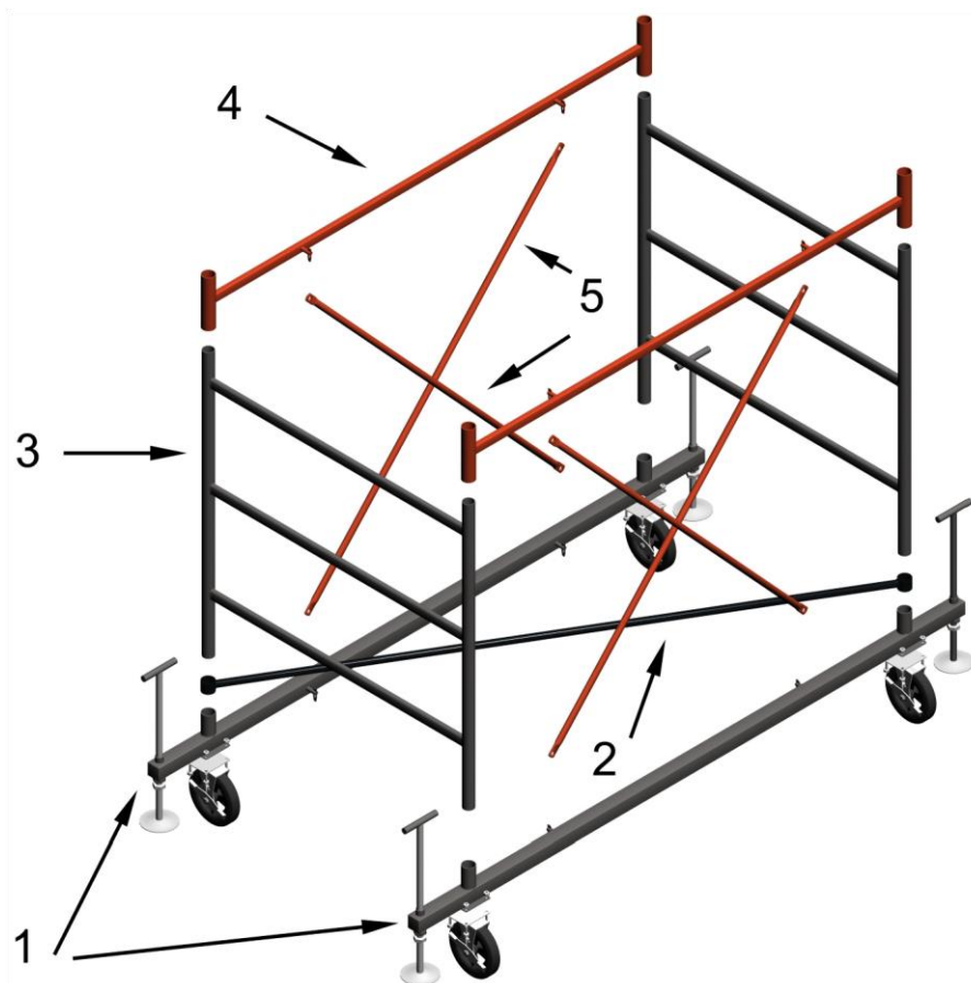
1. Балка базового блока 3. Лестница секции 5. Стяжка секц.
